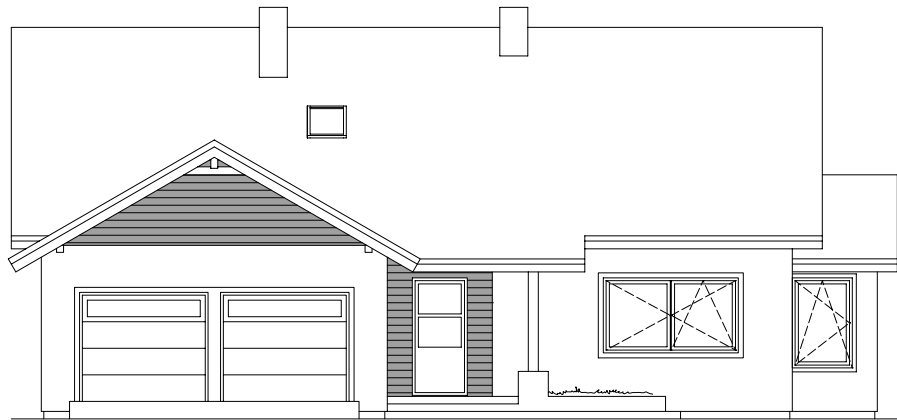
ELEWACJA FRONTOWA
